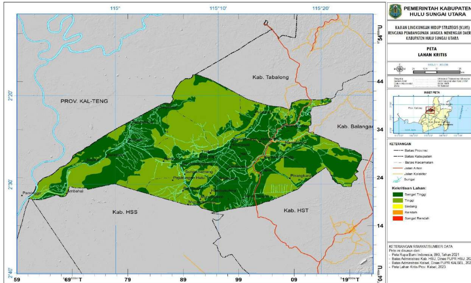
Gambar 2.14. Lahan Kritis Kabupaten Hulu Sungai Utara
