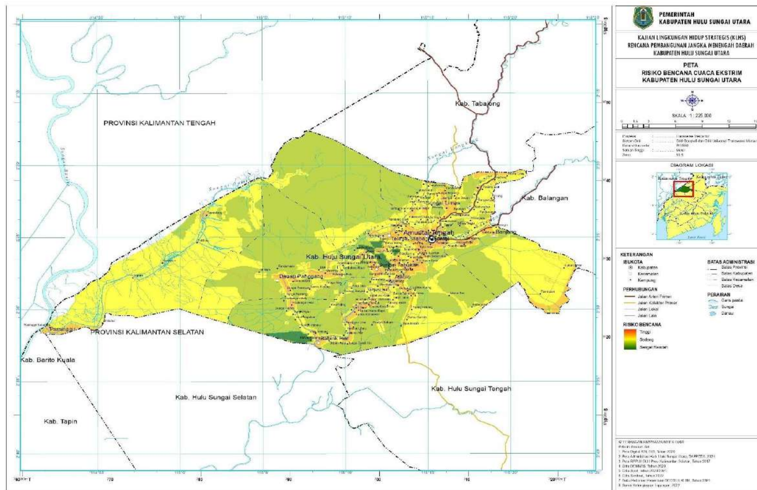
Gambar 2.12. Risiko Cuaca Ekstrem di Kabupaten Hulu Sungai Utara
