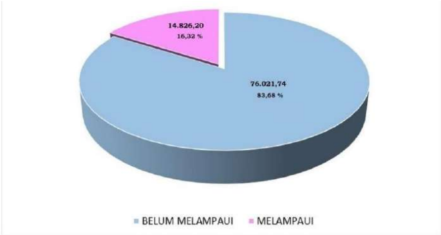
Gambar 2.4. Proporsi Daya Dukung Air Menurut DDDT Air Nasional
