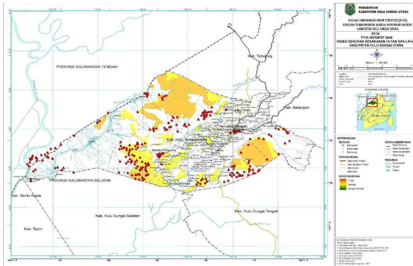
Gambar 2.11. Risiko Karhutla Kabupaten Hulu Sungai Utara
